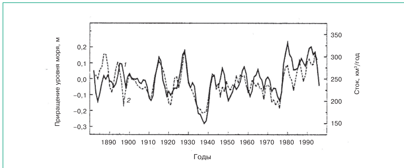
Рис. ТР10.3. Приращение уровня Каспийского моря за год (1, левая ось ординат) и годовой сток Волги (2, правая ось ординат).
