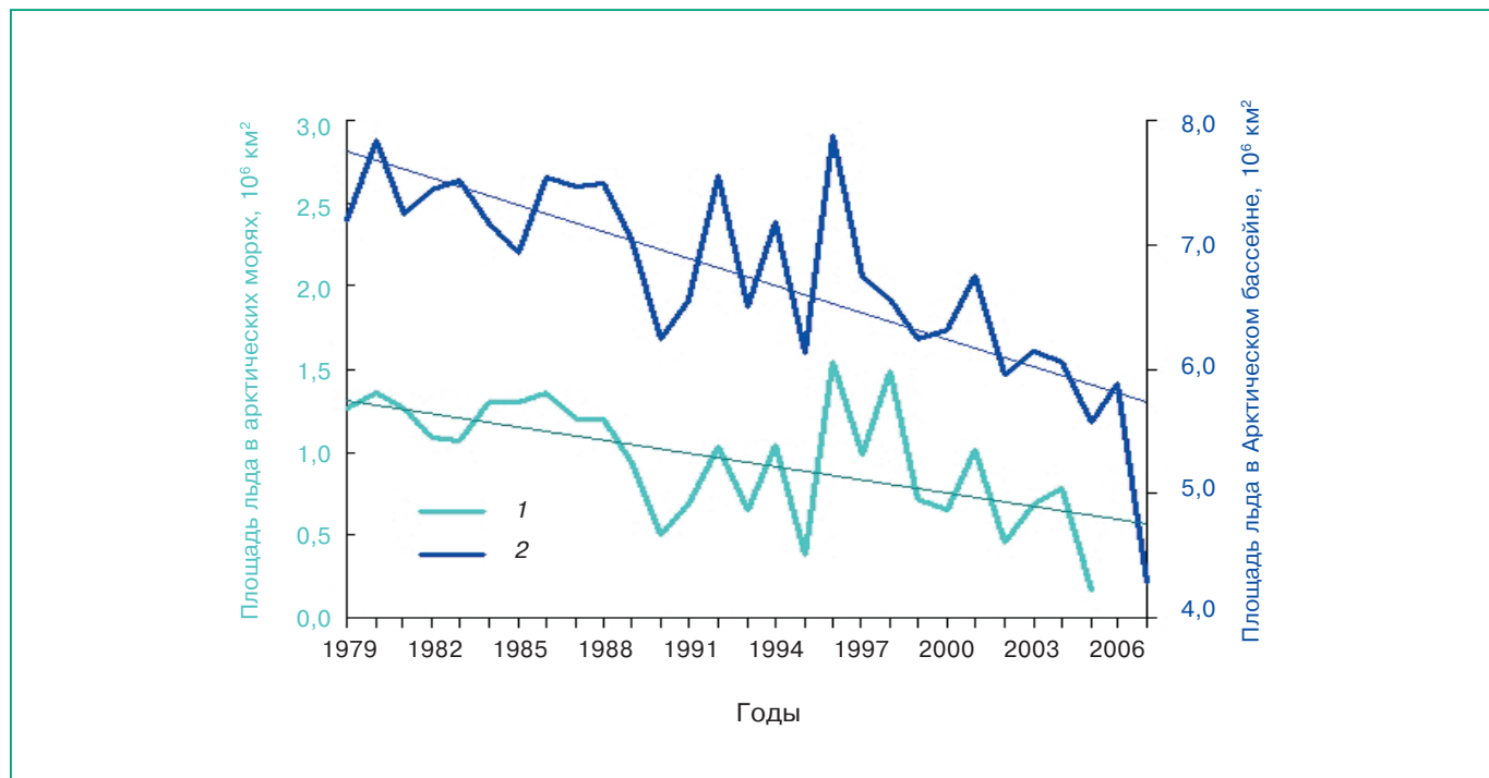
Рис. ТР3.4. Площадь морского льда в сибирских арктических морях (Карское, Лаптевых, Восточно-Сибирское и Чукотское) по данным ААНИИ (1) и в Северном полушарии по данным NSIDC (2) в сентябре за период 1979–2007 гг.
