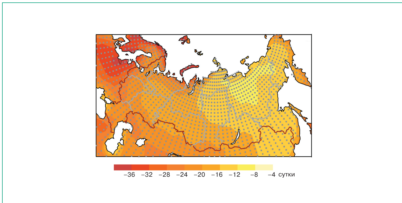
Рис. TP7.3. Уменьшение числа суток с морозом в году к середине XXI века по ансамблю из 9 МОЦАО для сценария А2. Точками обозначены узлы сетки, в которых средние изменения числа суток с морозом по ансамблю больше, чем средний межмодельный разброс.
