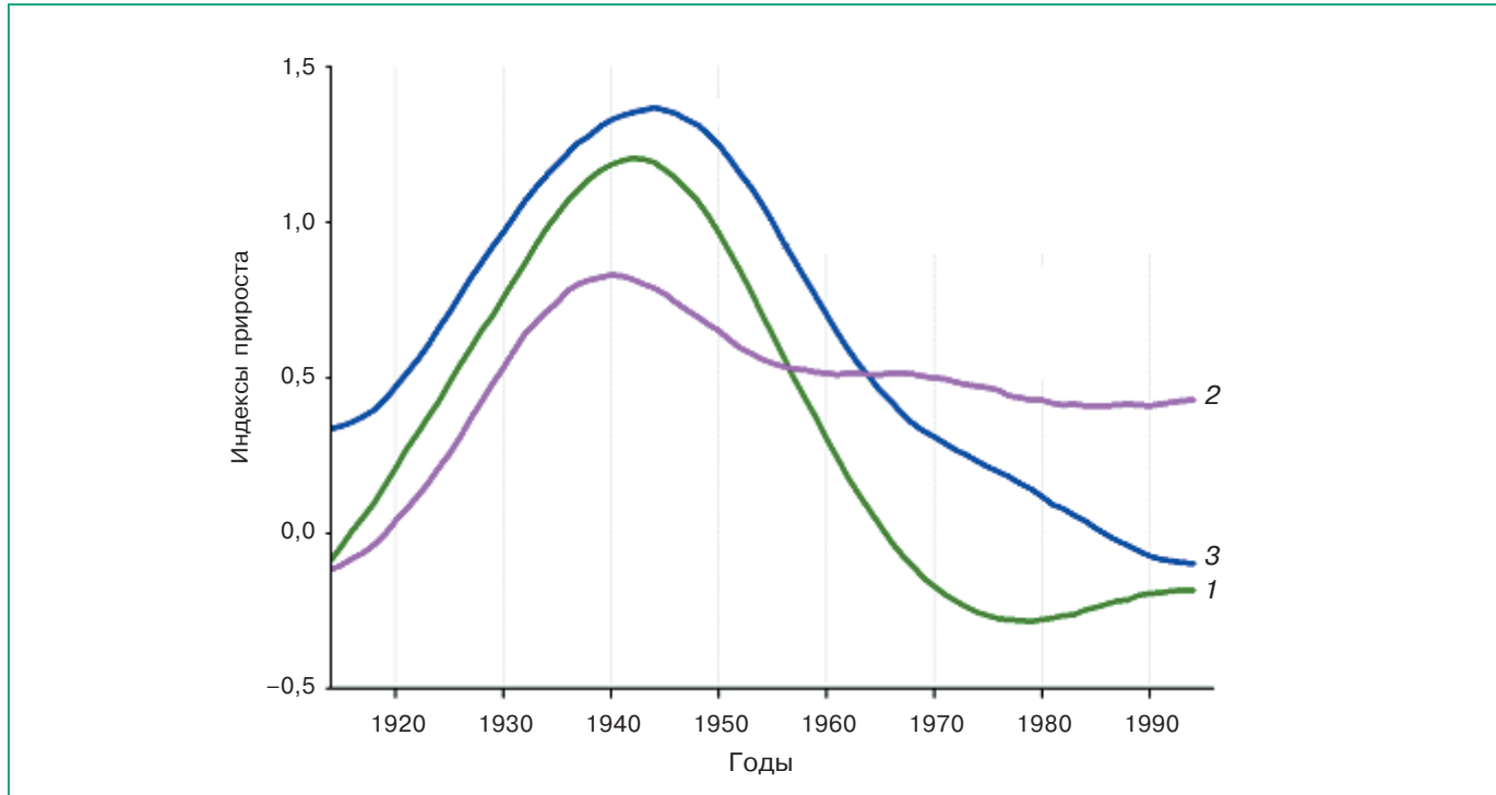
Рис. TP8.2. Индексы радиального прироста лиственницы, произрастающей на полярной (Таймыр (1) и Индигирка (2)) и верхней (в горах Тувы (3)) границах ареала на севере и юге Сибири соответственно.
