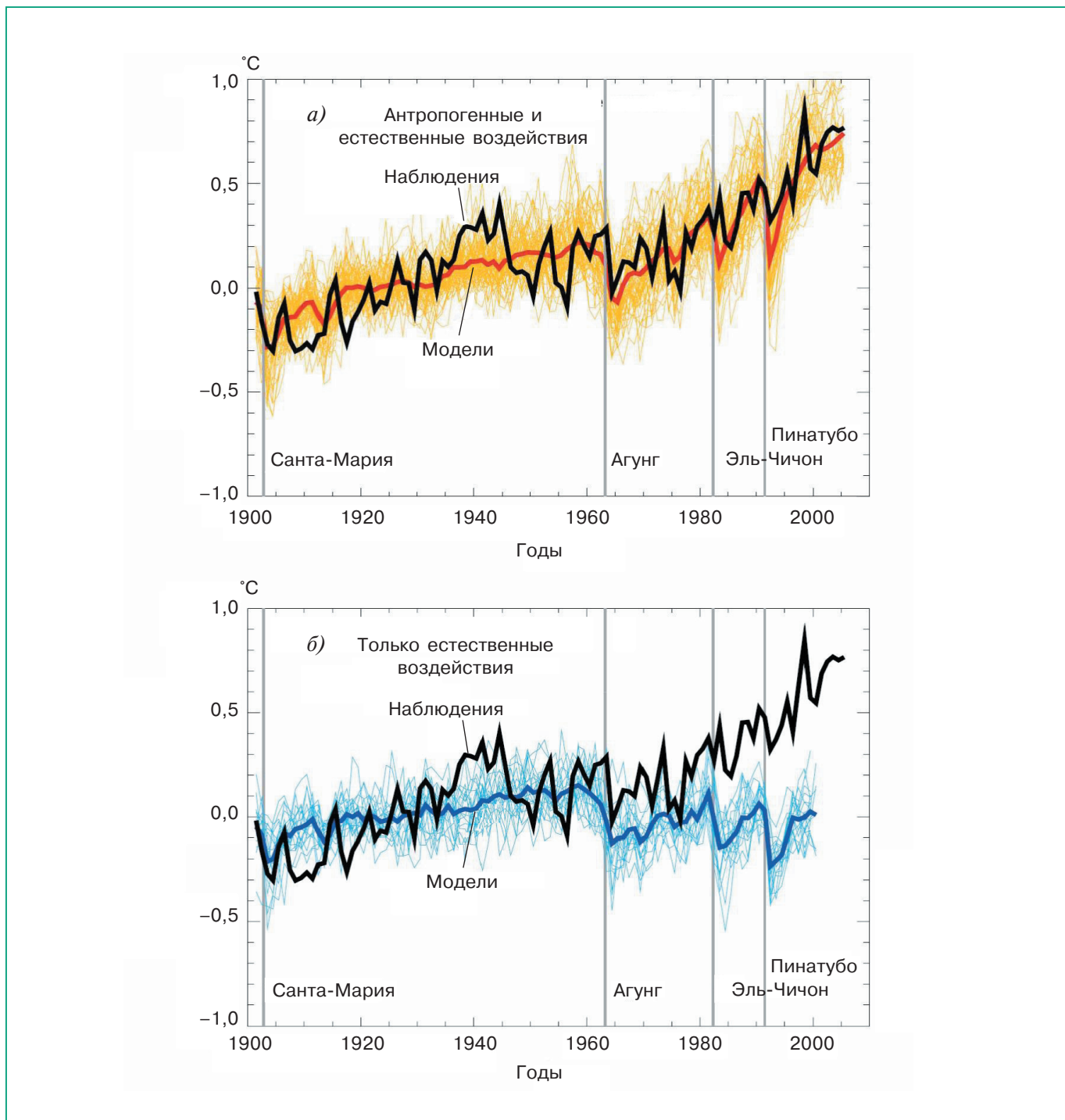
Рис. TP6.1. Аномалии средней глобальной температуры приземного воздуха (°C) по данным наблюдений и расчетов с учетом антропогенных и естественных внешних воздействий (а) и только естественных воздействий (б). К естественным воздействиям относятся изменения приходящего на верхнюю границу атмосферы солнечного излучения и влияние вулканической деятельности на аэрозольный состав атмосферы, а к антропогенным — изменения концентрации парниковых газов и сульфатного аэрозоля. Аномалии рассчитаны по отношению к среднему за 1901–1950 гг. На рисунке а результаты 58 расчетов по 14 МОЦАО показаны тонкими желтыми линиями, а среднее по мультимодельному ансамблю — жирной красной линией. На рисунке б представлены результаты 19 расчетов по 5 моделям. Расчеты показаны тонкими голубыми линиями, а среднее по мультимодельному ансамблю — жирной синей линией. Серыми линиями отмечено время наиболее значительных извержений вулканов.
