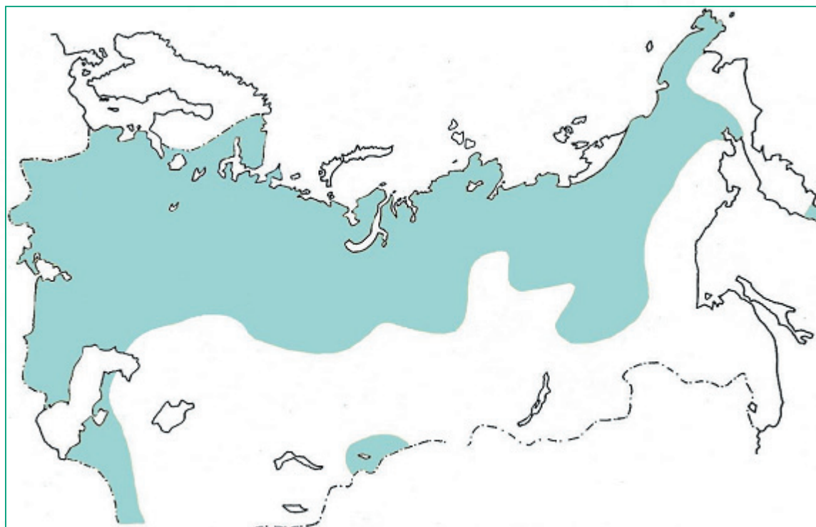
Рис. TP12.1. Тренды испаряемости в 1949–1990 гг. на территории бывшего СССР. Голубым цветом выделена область отрицательных трендов; на остальной части территории тренды положительные или отсутствуют.
