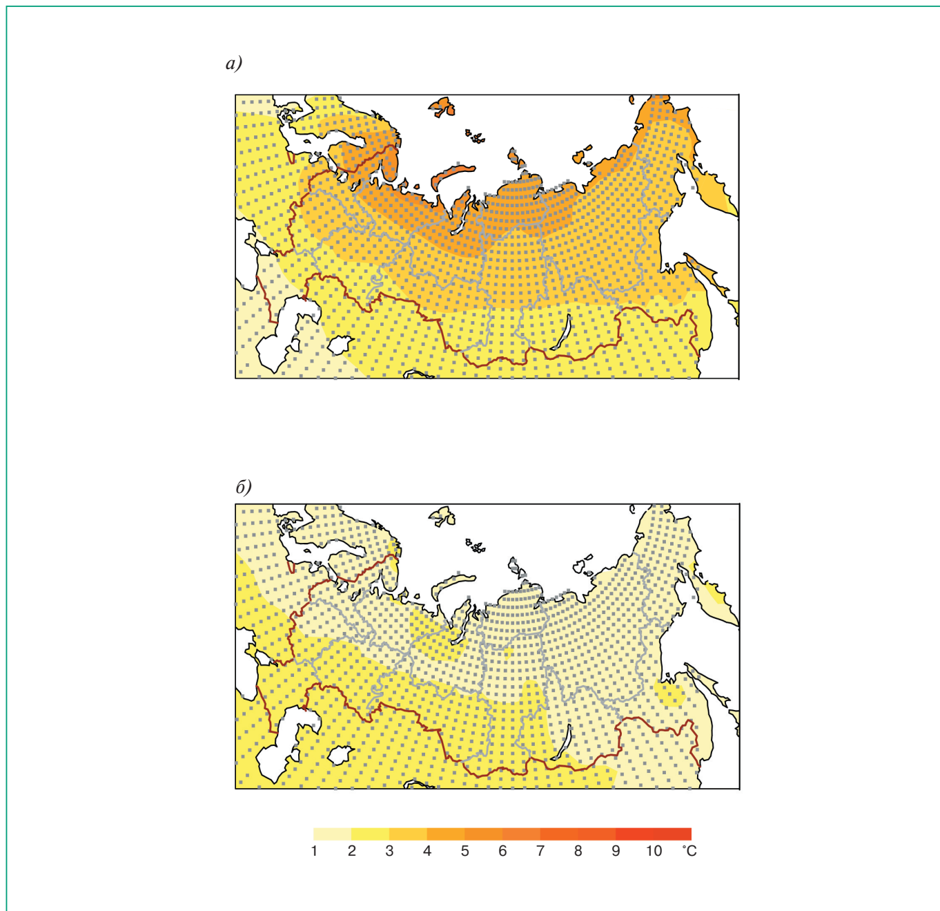
Рис. ТР7.2. Изменения температуры приземного воздуха (°С) на территории России зимой (а) и летом (б) в середине XXI века (2041–2060 гг.), рассчитанные по ансамблю МОЦАО СМIP3 для сценария А2. Точками обозначены области, в которых средние изменения температуры воздуха по ансамблю превышают стандартные отклонения межмодельного разброса (т. е. сигнал больше шума).
