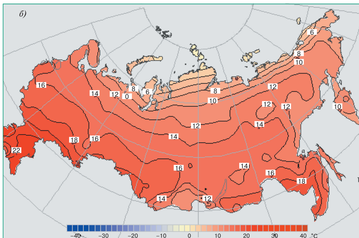
Рис. ТР1.2. Средняя температура приземного воздуха (°C) зимой (а) и летом (б) за период 1961–1990 гг.
