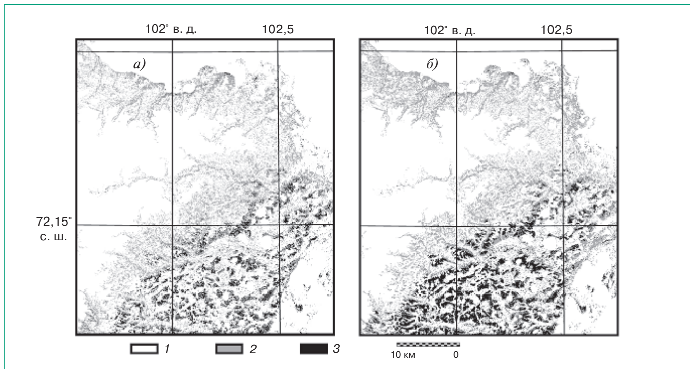
Рис. TP8.3. Снимки урочища Ары-Мас. а — 1973 г.; б — 2000 г.; 1 — фон (тундра и пойма реки), 2 — редины и редколесья (сомкнутость крон < 0,3), 3 — древостои (сомкнутость крон ≥ 0,3).
