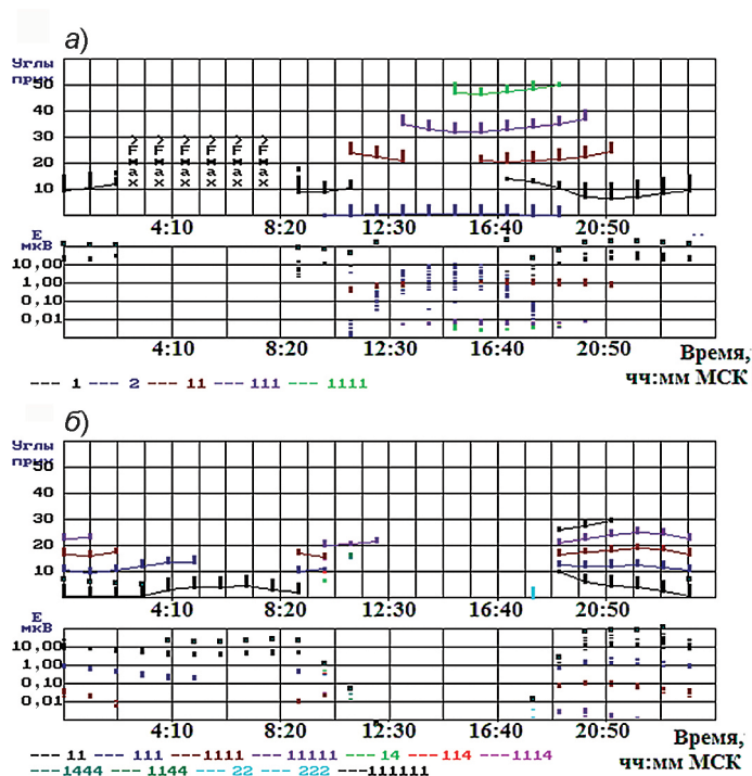
Рис. 3. Результаты моделирования углов места и уровня напряженности суммарного и отдельных модов КВ-радиосигнала в месте приема на трассах «Лондон — Север Норвегии» (а) и «Лондон — Дуала (Африка)» (б).
