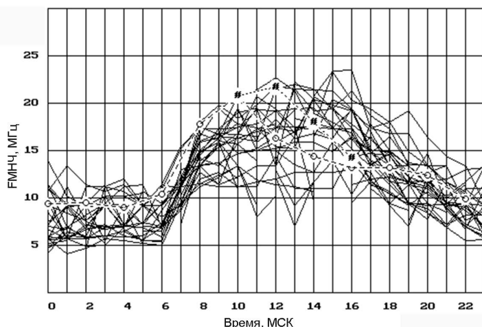
Рис. 2. Результаты экспериментально измеренных методом наклонного зондирования ионосферы ( — ) и рассчитанных по модели КВ-радиоканала (--o--, ·#·) значений максимально наблюдаемых частот на трассе Москва — станция «Северный полюс», 15 октября 1975 г.
