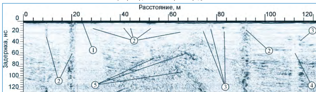
Пример типичного временного георадарного разреза, выполненного при лоцировании зон трещин в ледовом массиве: 1 – нулевая отметка (поверхность ледника); 2 – отражения от стенок приповерхностных трещин; 3 – отражения от стенок широких трещин, перекрытых относительно мощными снежными мостами; 4 – отражения, характеризующиеся значимым ослаблением сигнала, связанные с затуханием волн в трещине; 5 – отражения, связанные с инородными включениями (например, обломков горных пород).
