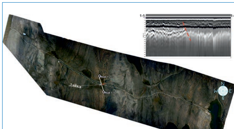
Рис. 5. Ортофотоплан и георадарный профиль в районе залива Медвежий. Разломная зона указана пунктиром
