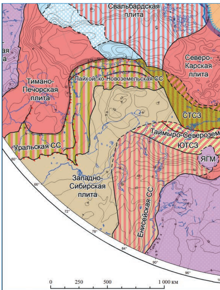
Рис. 3. Фрагмент схемы фундамента АЗРФ
