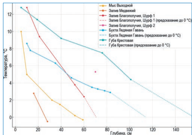
Рис. 11. Зависимость температуры грунта от глубины с предположительными данными начала распространения многолетней мерзлоты
