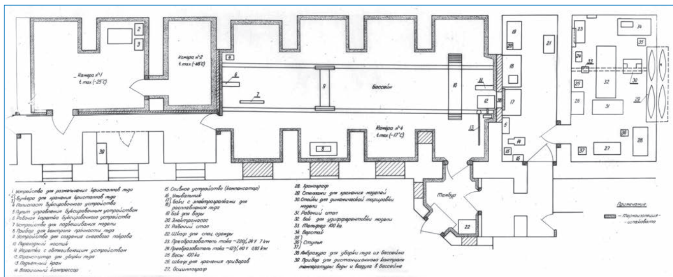
Рис. 3. Схема расположения части ледоисследовательской лаборатории с ледовым бассейном (рисунок 1958 года)
