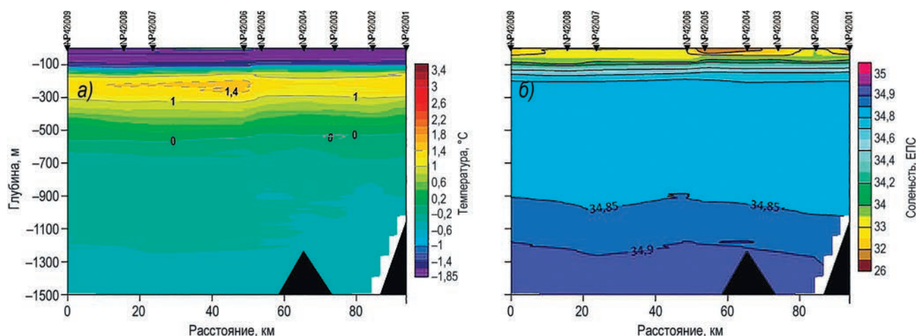
Распределение температуры воды, °C (а) и солёности, ЕПС (б) на квазизональном разрезе через южную часть хребта Ломоносова
