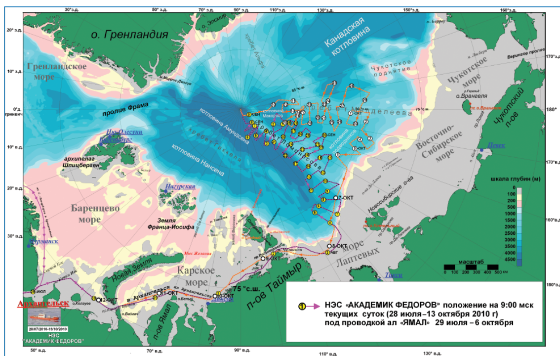
Схема маршрута 31-го рейса НЭС «Академик Федоров»
